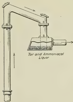
FIG. 58.—Hydraulic Main.
